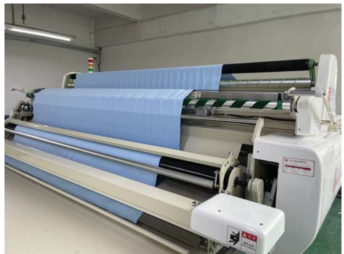
自动裁床
